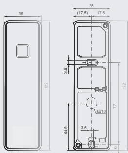
dormakaba Erfassungseinheit 90 04, Standard-Ausführung
