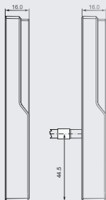
dormakaba Erfassungseinheit 90 04, Seitenansicht mit Kabelabgang
