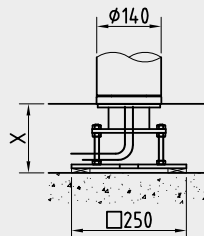
Mit Trägerplatte auf Rohfußboden
